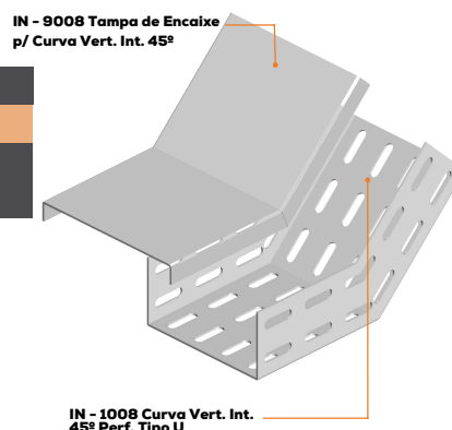
IN - 1008 Curva Vert. Int. 45° Perf. Tipo U
